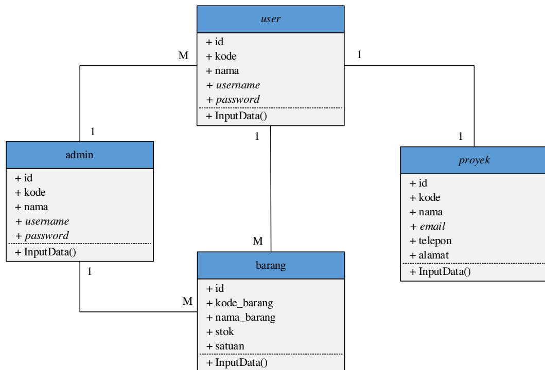
Gambar 8. Class Diagram Sistem Informasi Manajemen Inventaris
