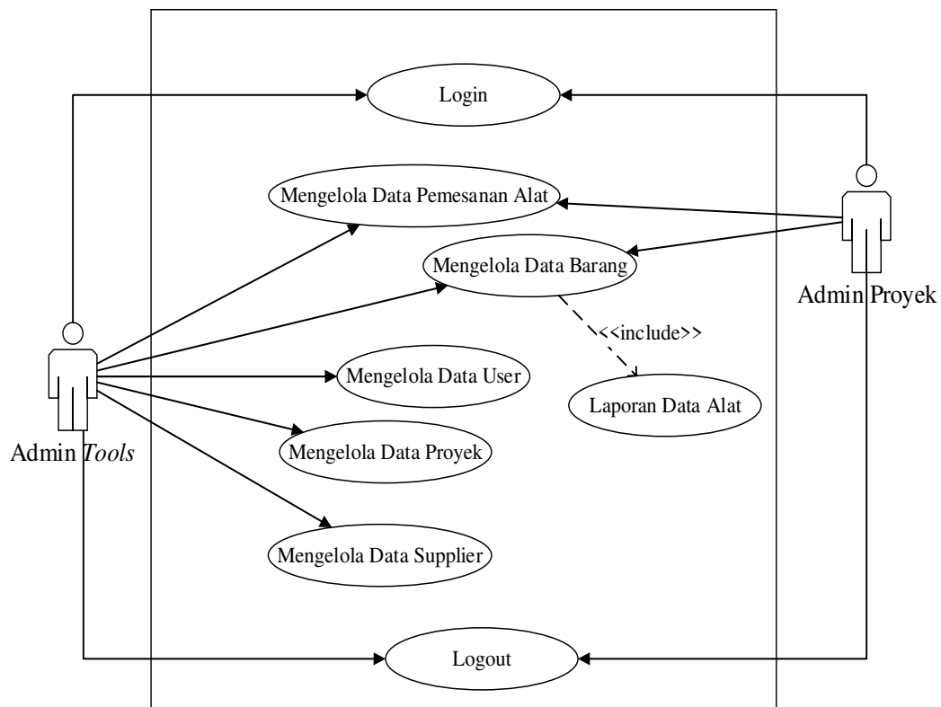
Gambar 2. Use case diagram sistem informasi manajemen inventory
