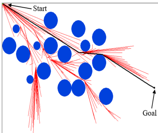
Gambar 11. Bentuk pohon pencarian pada metode hybrid sampling pada lingkungan clutter
