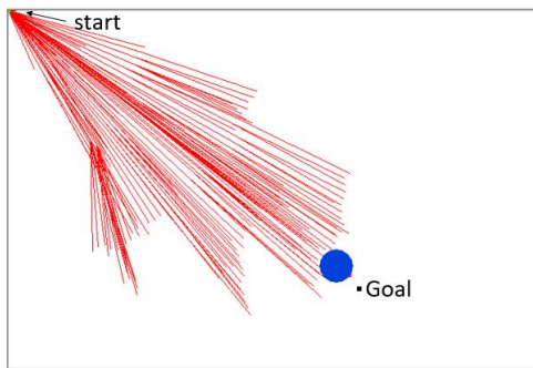
Gambar 4. Pohon pencarian pada kondisi titik tujuan membelakangi obstacle menggunakan boundary sampling
