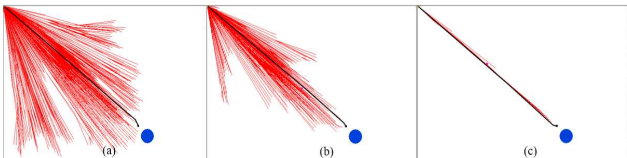
Gambar 2. Perbandingan pohon pencarian pada kondisi titik tujuan berada di dekat obstacle dan berhadapan langsung dengan titik awal: random sampling (a), goal biasing sampling (b), boundary sampling (c).
