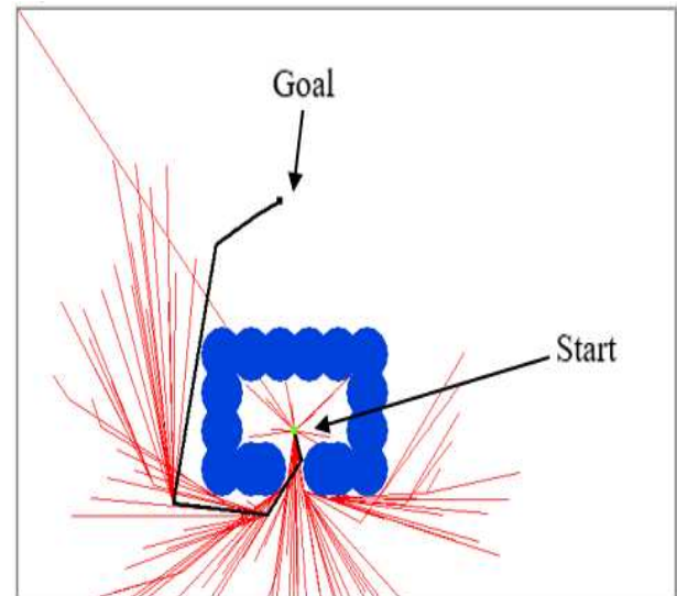
Gambar 15 bentuk pohon pencarian pada metode hybrid sampling dilingkungan trap
