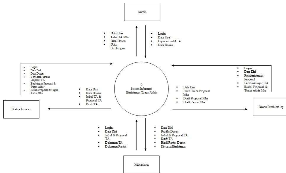
Gambar 1. Diagram konteks
