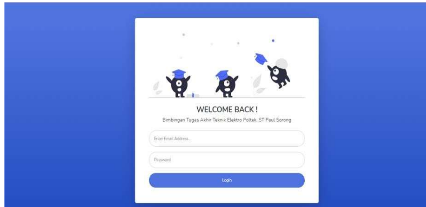
Gambar 3. Login
