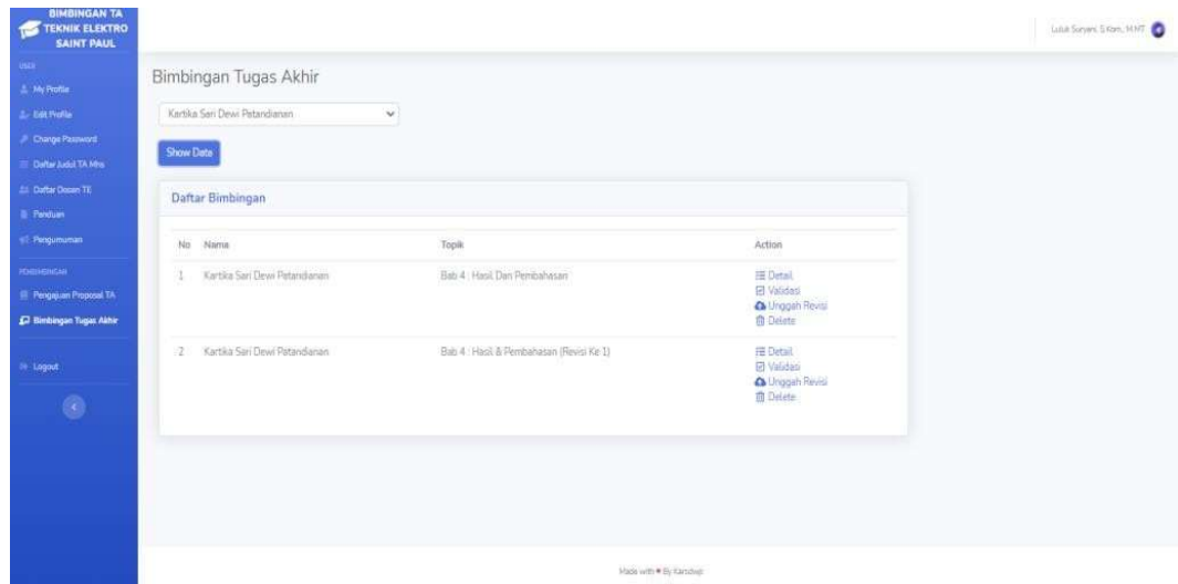
Gambar 7. Bimbingan TA.
