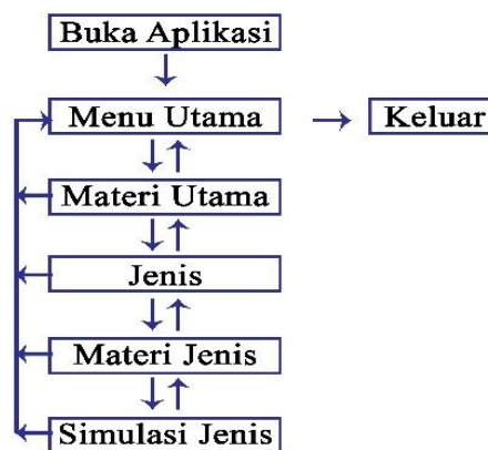
Gambar 3 Flowchart Aplikasi
