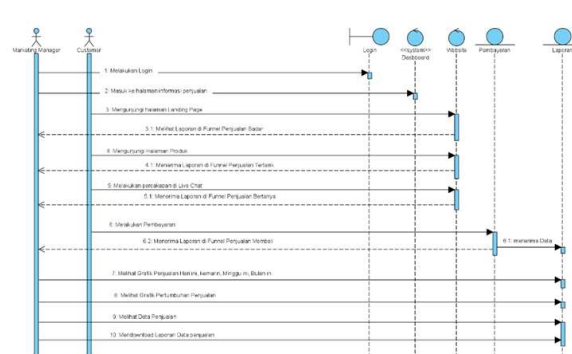
Gambar 4 Sequence Diagram yang diusulkan
