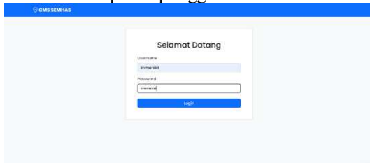
Gambar. 8 Halaman Login
