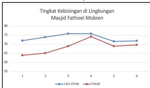
Gambar 4. Tingkat Kebisingan di Masjid Raya Fathoel Mobien
