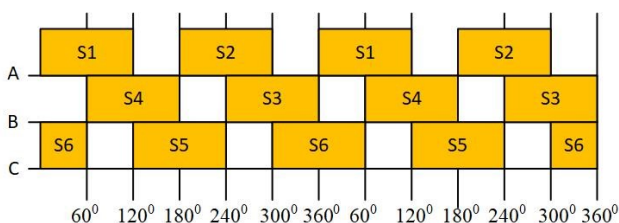
Gambar 3: Gelombang Komutasi 120^\circ
