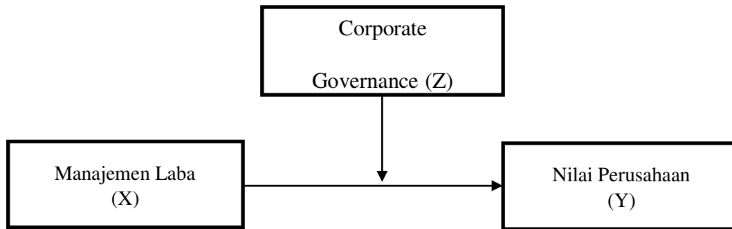
Gambar 2. Kerangka Teoritis
