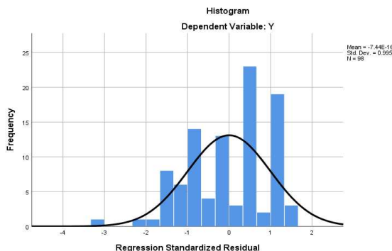
Gambar 1. Diagram Histogram Untuk Uji Normalitas
