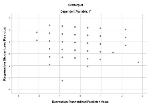
Gambar 2. Uji Heteroskedastisitas Melalui Diagram Scatterplot
