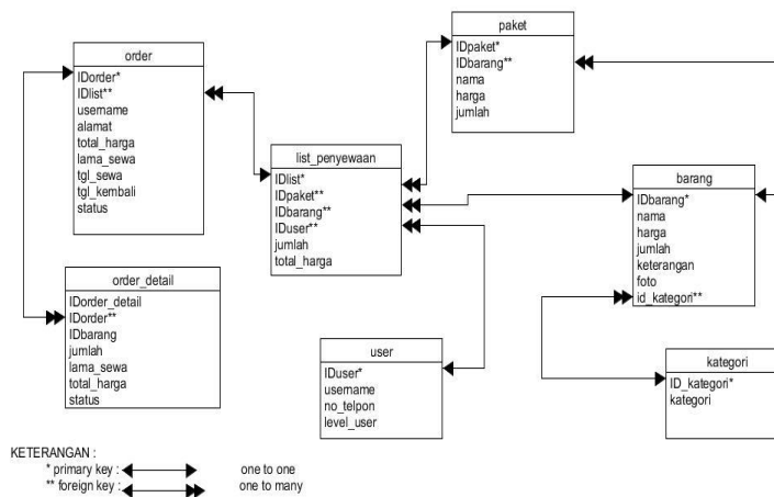
Gambar 3.7 Relasi Tabel
