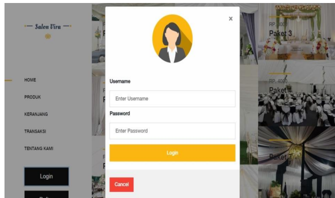
Gambar 4.7 Halaman Login
