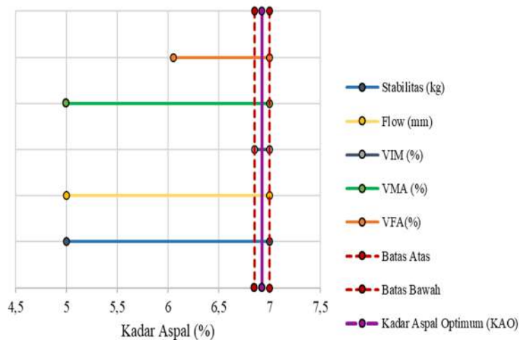
Fig 1. Optimum Asphalt Content Chart (KAO)
