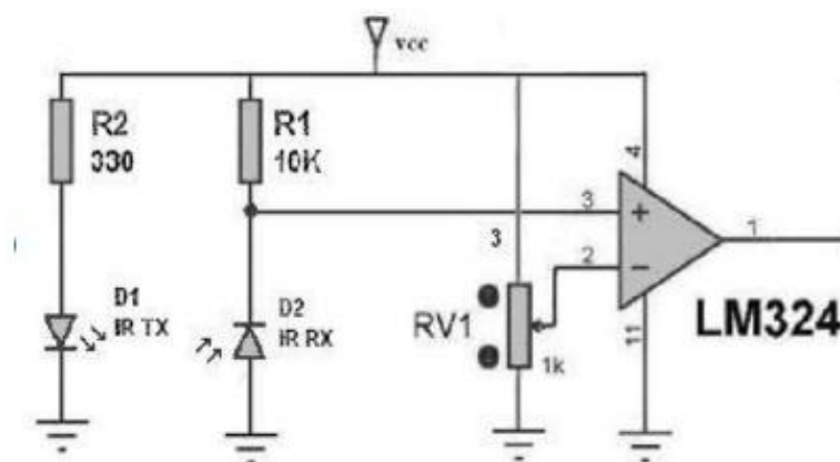
Gambar 4. Skematik Rangkaian IR Obstacle sensor [10].
