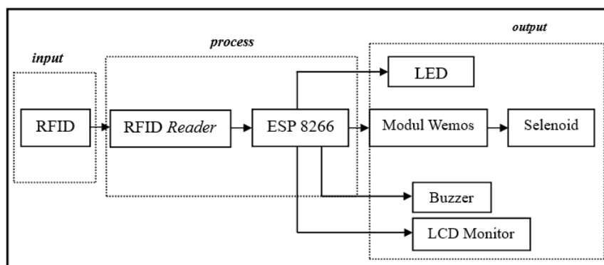
Gambar 2. Diagram Blok Rangkaian Pintu Otomatis
