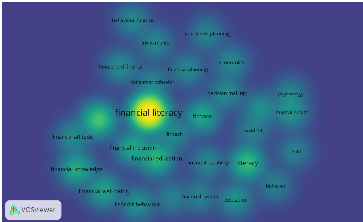
Gambar 3. Visualisasi Densitas
