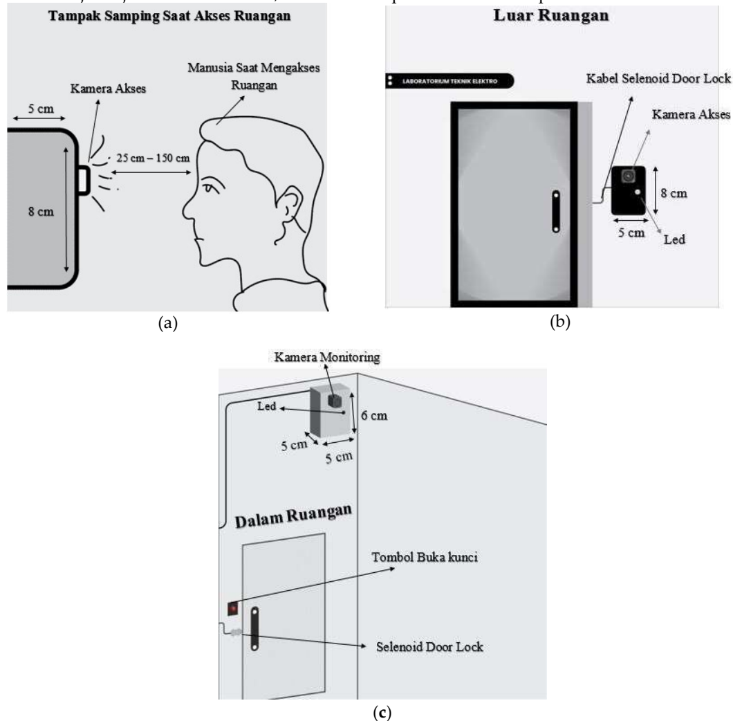
Gambar 5. Rencana penempatan sistem: (a) Kamera akses tampak samping; (b) Kamera akses ditempatkan di depan pintu laboratorium; (c) Kamera monitoring, selenoid door lock, dan tombol buka kunci dari dalam ruangan laboratorium.
