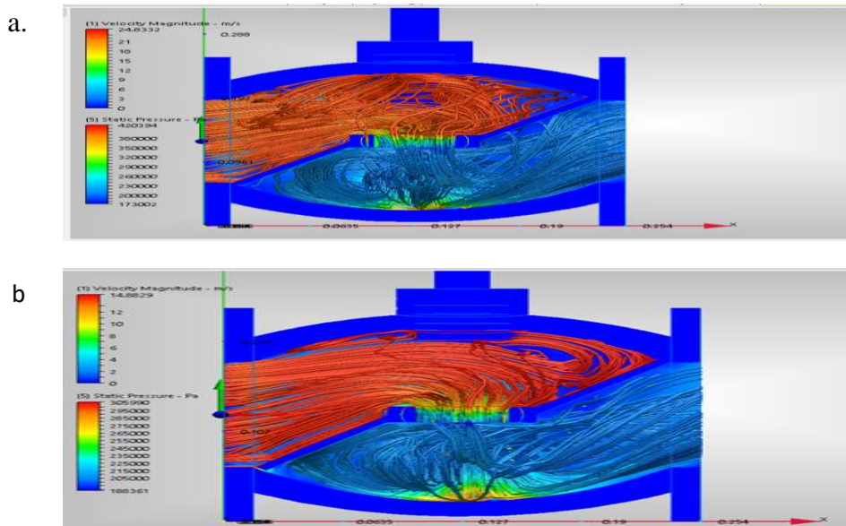
Gambar 3.4 counter distribusi a. bukaan valve 50 % dengan tekanan 4 bar
