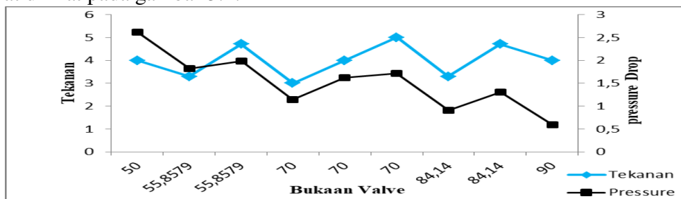
Gambar 3.1 Pengaruh bukaan valve dan tekanan terhadap pressure drop
