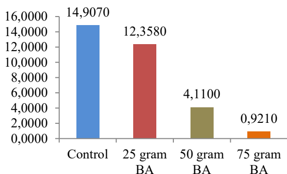
Gambar 2. Hasil Pengujian Parameter TSS Menggunakan Adsorben Bottom Ash
