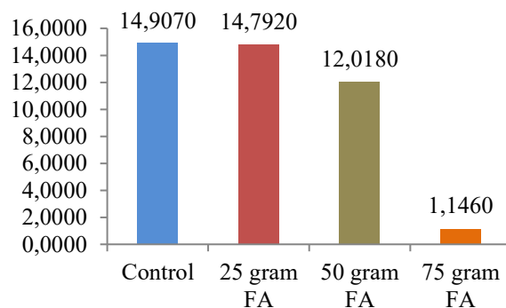
Gambar 1. Hasil Pengujian Parameter TSS Menggunakan Adsorben Fly Ash
