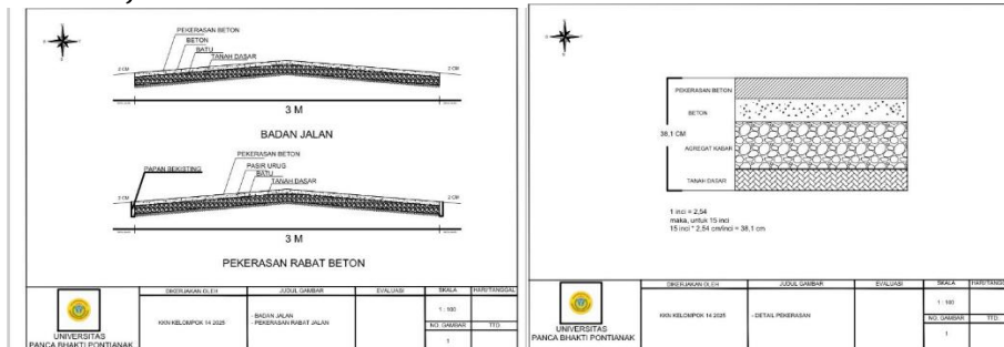
Gambar 6. dokumen teknis pembangunan jalan beton
