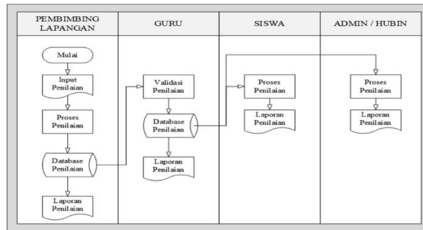
Gambar 1. Flowchart Pelaporan OJT
