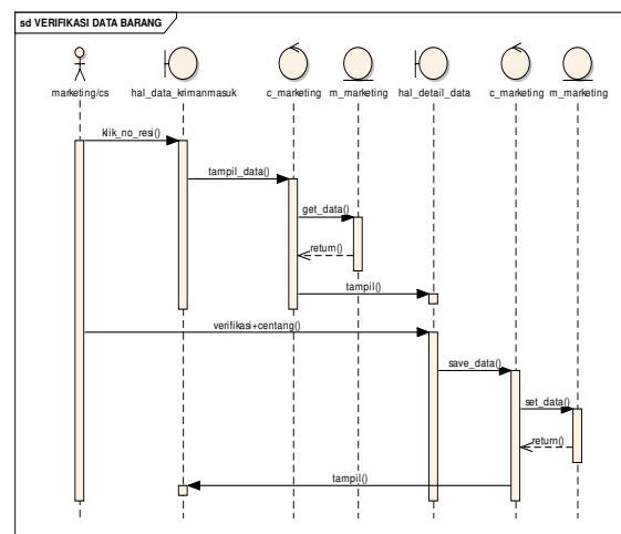
Gambar 4. Sequence Diagram Verifikasi Data Barang
