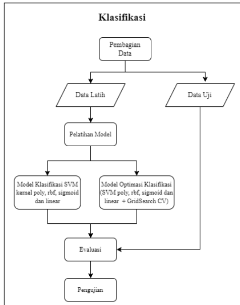
Gambar 2. Alur Klasifikasi
