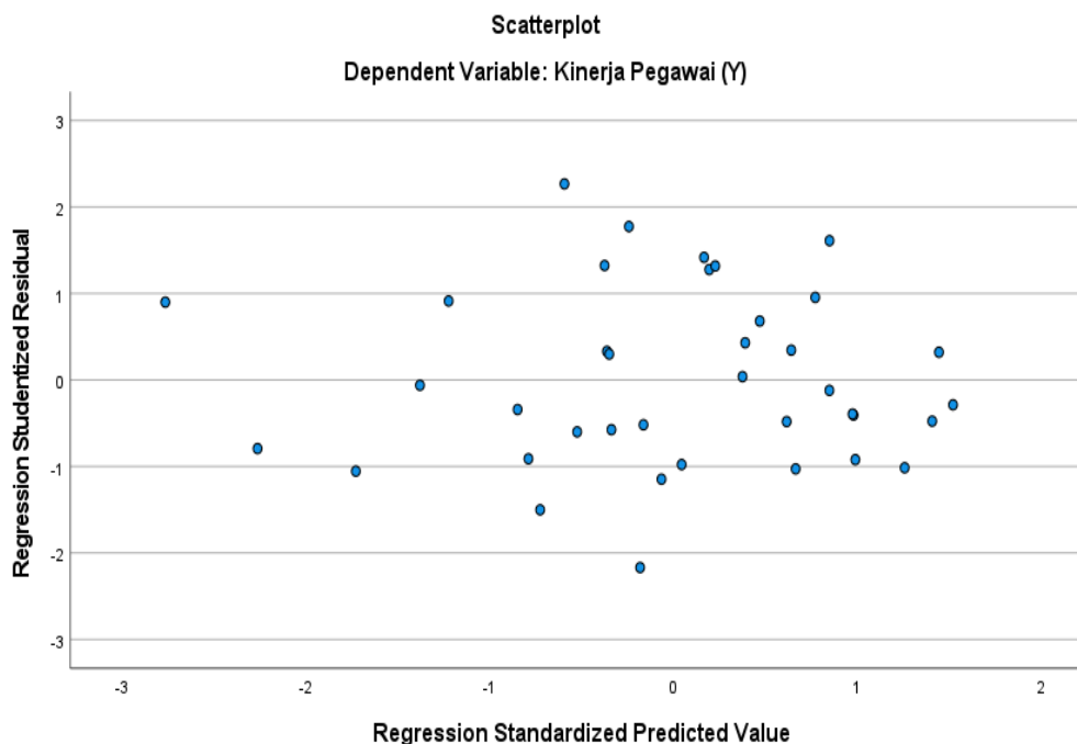
Gambar 4.2. Uji Heteroskedasitas
