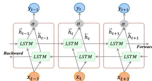
GAMBAR 1. Struktur BiLSTM
