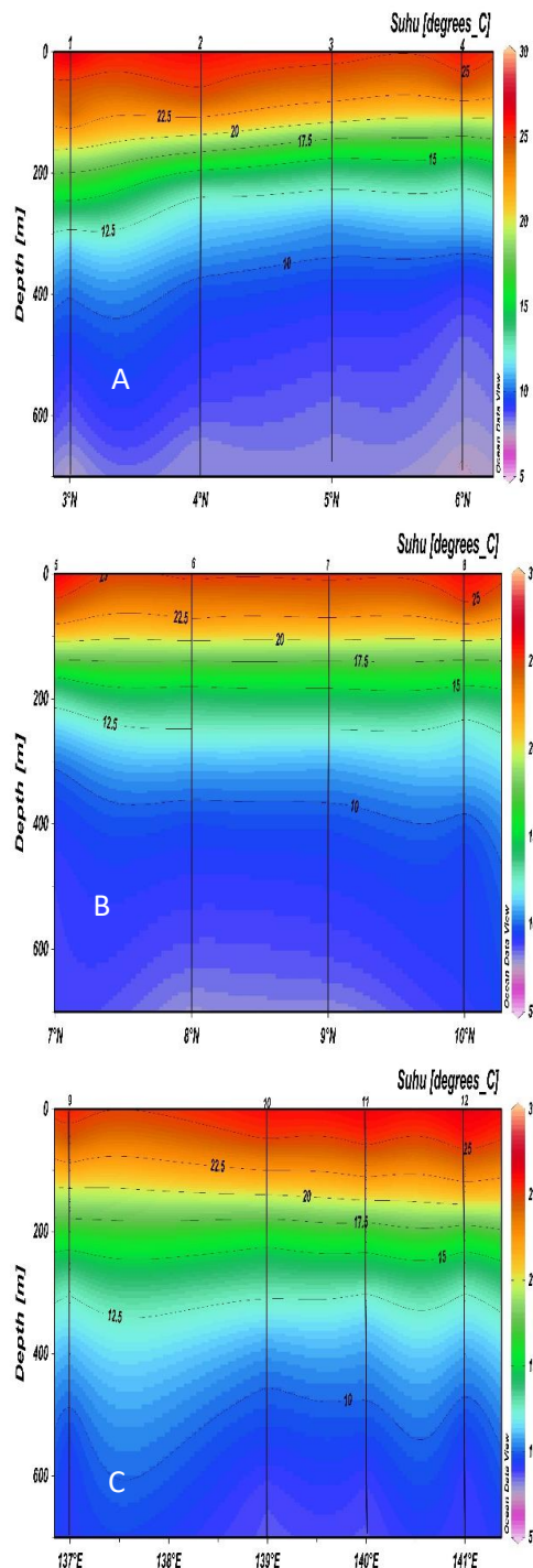
Gambar 2. Sebaran Melintang Suhu pada transek penelitian (a) Transek A, (b) Transek B, dan Transek C
