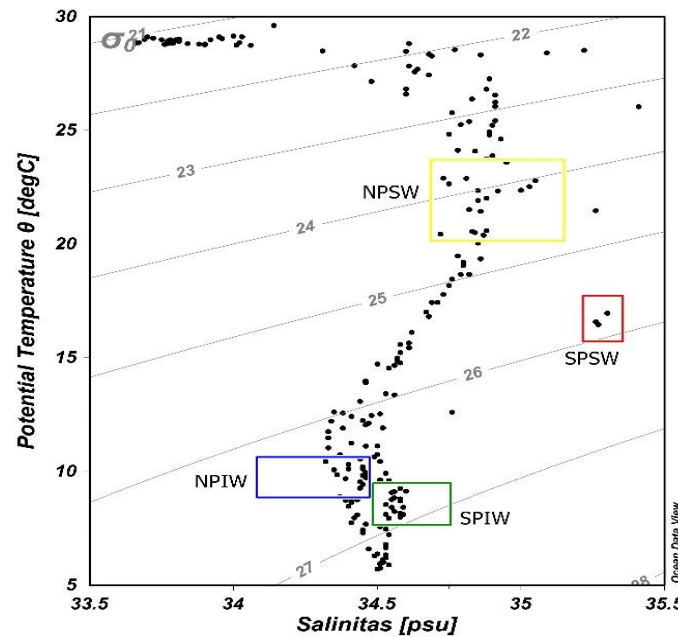
Gambar 4. Diagram T-S untuk semua stasiun pengamatan.
