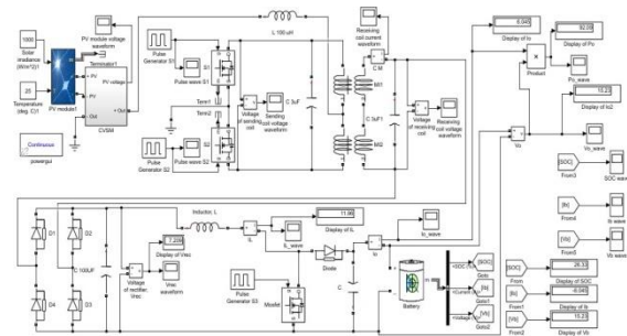
Gambar 2. Pemodelan Sistem Transfer Daya Fotovoltaik Nirkabel Untuk Sistem Pengisian Baterai
