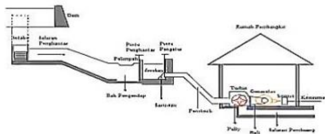
Gambar 1 Model Perencanaan PLTMH (Murtadlo, 2021)
