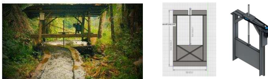
Gambar 5 Kondisi PTMH Desa Kalianan dan Desain Pintu air Otomatis (Setiyoko et al., 2025; Widodo et al., 2025)
