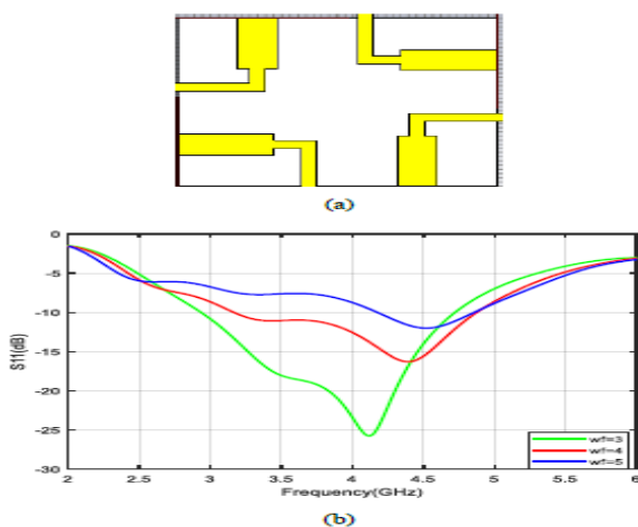
Gambar 11. Ukuran Feedline ( W_f ) (a). Desain W_f setelah dioptimasi, (b). Hasil simulasi Feedline ( W_f )
