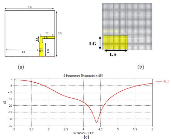
Gambar 5. Desain antenna dengan penambahan groundplane yang berbentuk kotak vertikal (a). Single patch , (b). Groundplane , (c). Hasil simulasi S11
