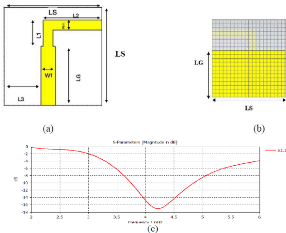
Gambar 3. Desain antenna dengan ukuran substrate 20 x 20 mm a. Single Patch , b. Groundplane , c. Hasil simulasi S11
