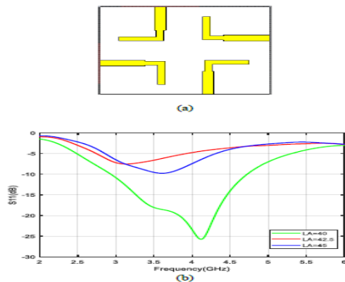
Gambar 10. Ukuran Substrate ( L_s ) (a). Desain ( L_s ) setelah dioptimasi, (b). Hasil simulasi ( L_s )
