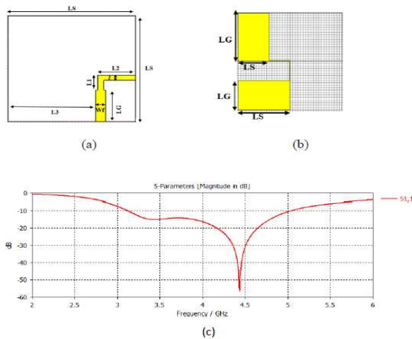
Gambar 7. Desain antenna dengan penambahan pada groundplane dengan 4 elemen sisi patch (a). Single patch , (b). Groundplane , (c). Hasil simulasi S11
