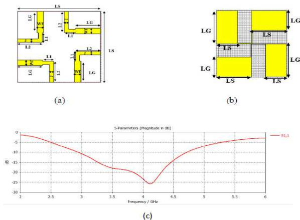
Gambar 8. Desain antenna dengan menambahkan patch pada bagian masing-masing ground yang memiliki bentuk patch L terbalik (a). Desain antenna dengan empat patch (empat elemen), (b). Groundplane , (c). Hasil simulasi S11
