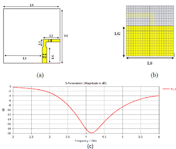
Gambar 4. Desain antenna dengan ukuran substrate 40 x 40 mm a. Single patch , b. Groundplane , c. Hasil simulasi S11
