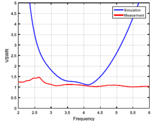
Gambar 16. Perbandingan VSWR
