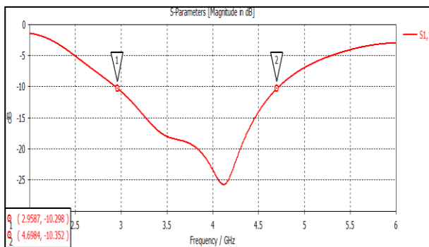
Gambar 14. Hasil return loss pada S11
