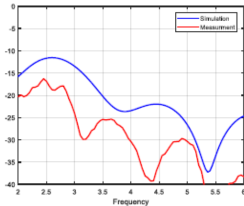
Gambar 17. Perbandingan Isolasi antara simulasi dan modifikasi
