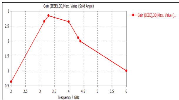
Gambar 13. Gain pada antenna referensi
