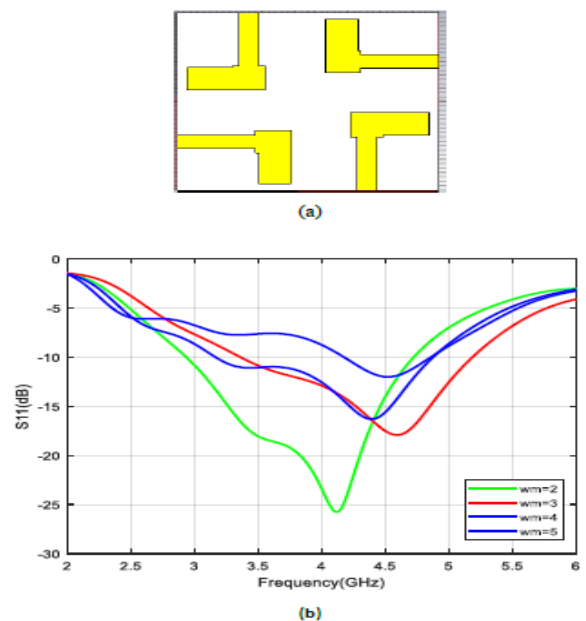
Gambar 9. Perbandingan Nilai Return Loss (a). Desain Patch ( W_m ) setelah di optimasi, (b). Hasil simulasi patch ( W_m )
