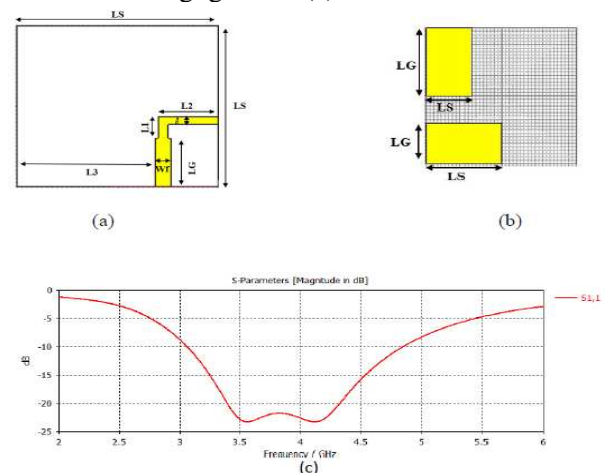
Gambar 6. Desain antenna dengan penggabungan antara dua groundplane (a). Single Patch , (b). Groundplane , (c). Hasil Simulasi S11
