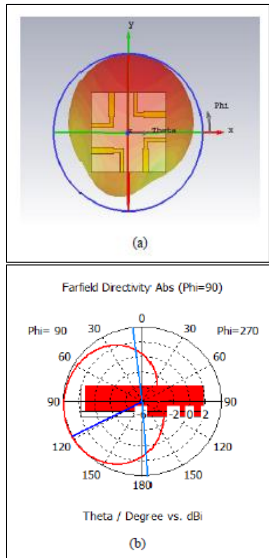
Gambar 12. Pola radiasi (a). Pola radiasi 3D, (b). Pola radiasi polar
