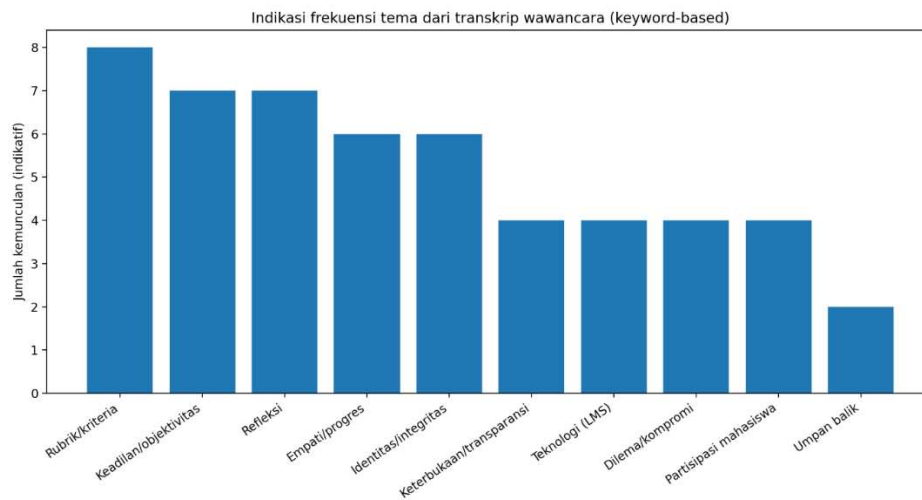
Gambar 1 Frekuensi Tema
