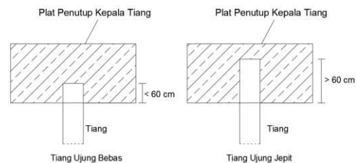
Gambar 2.6 Definisi Tiang Ujung Bebas dan Jepit (Sumber: Alihudien, A dan Proyono, P)
