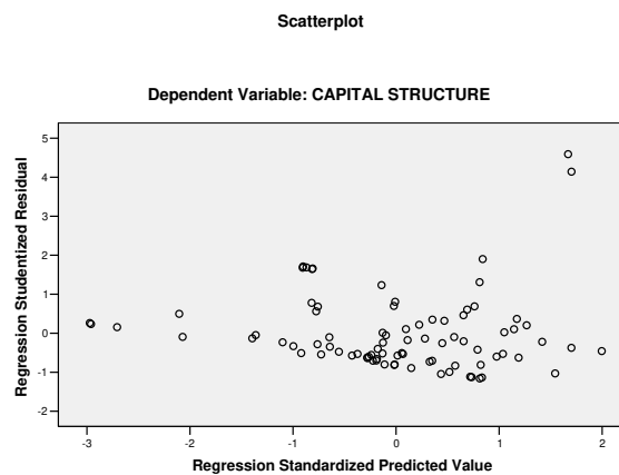
Gambar 2. Uji Heterokedastisitas – Grafik Scatterplot
