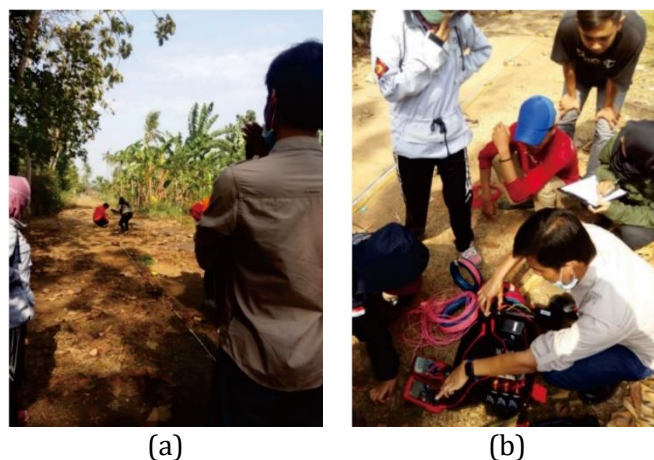
Gambar 6. Proses pengambilan data (a) anggota tim memantau penancapan elektroda pada tanah dan pemasangan kabel pada elektroda, serta (b) anggota tim melakukan pengukuran data menggunakan alat geolistrik
