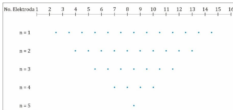
Gambar 5. Susunan 16 elektroda beserta representasi data yang diukur pada setiap nilai n (adopsi dari Djereng dkk., 2017)
