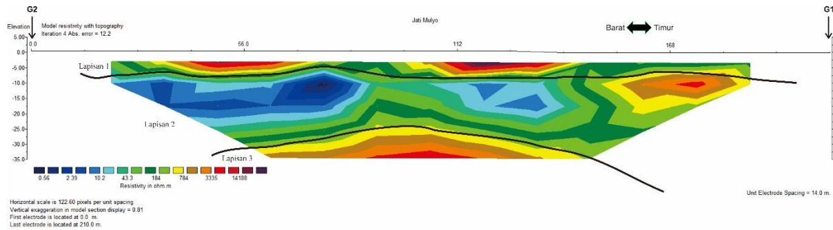
Gambar 7. Hasil pengolahan data menggunakan perangkat lunak Res2DInv.
