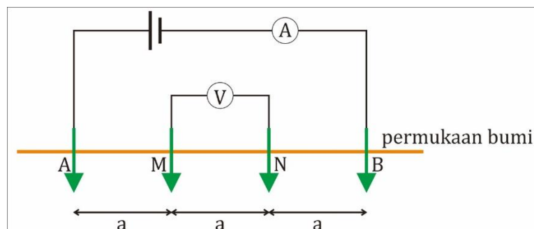
Gambar 3. Susunan elektroda dan alat ukur (A = Amperemeter dan V = Voltmeter ) dalam metode geolistrik (adopsi dari Manrulu et al., 2018; Sastrawan & Latifan, 2018)
