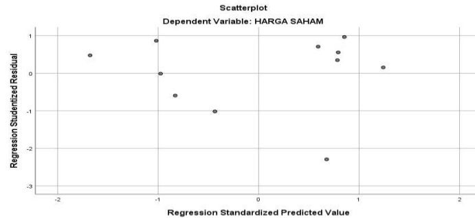
Gambar 1. Uji Heteroskedastisitas
