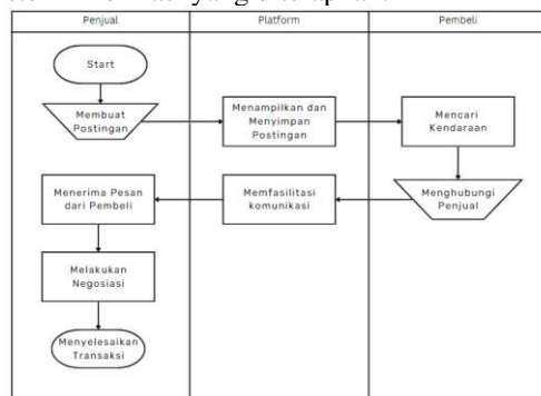
Gambar 2. Aliran Sistem Informasi Lama
