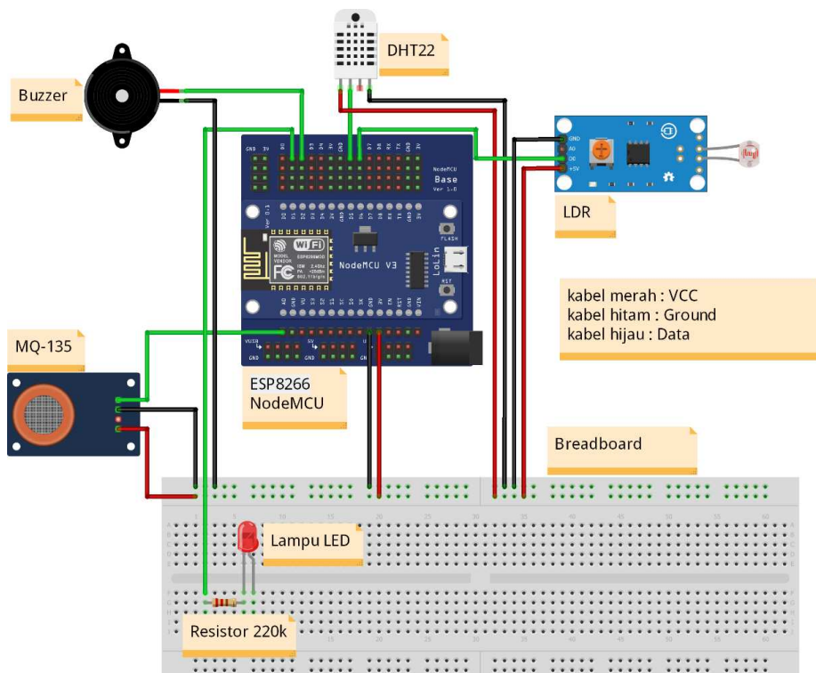
Gambar 2 Skematik rangkaian
