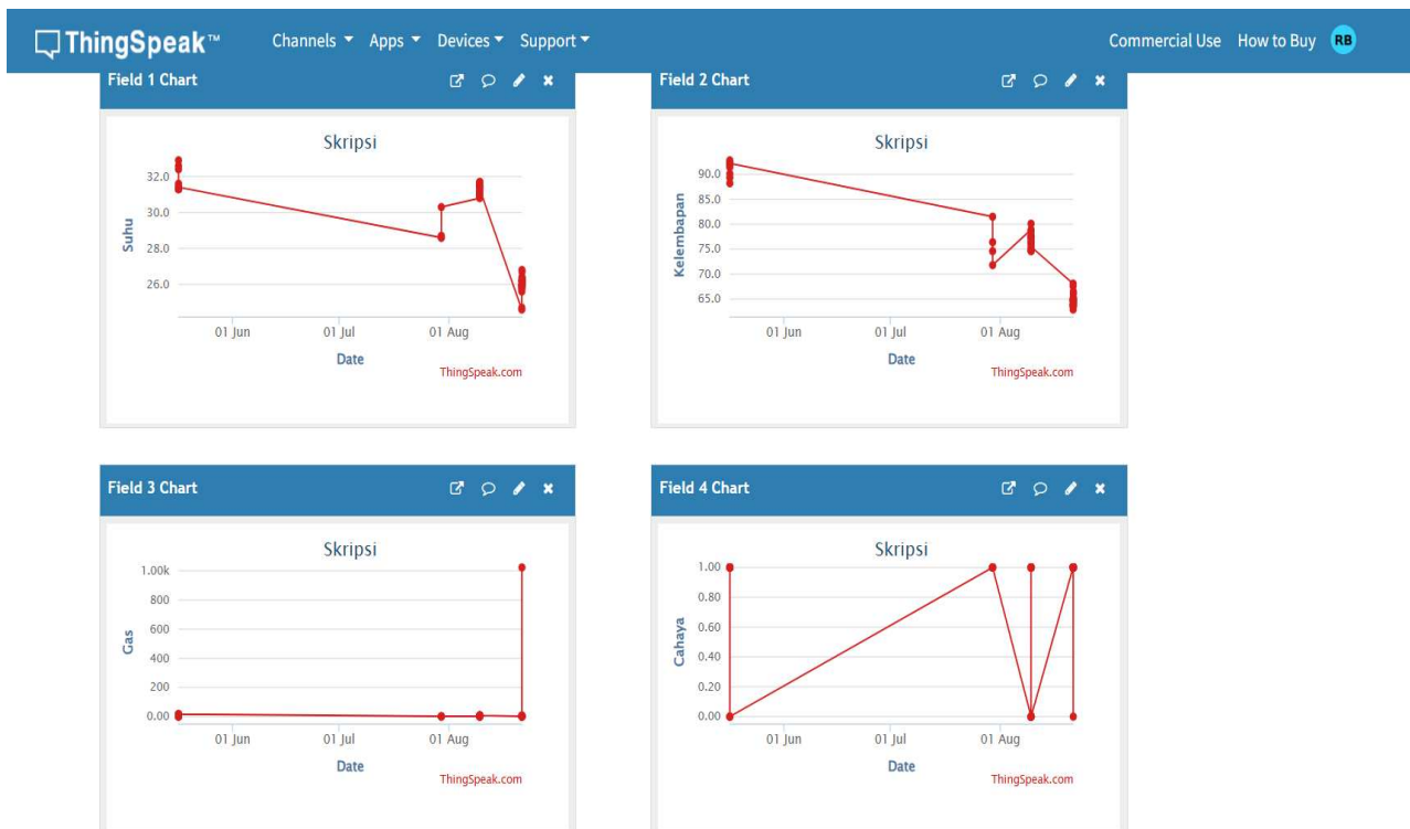
Gambar 4 Tampilan data
