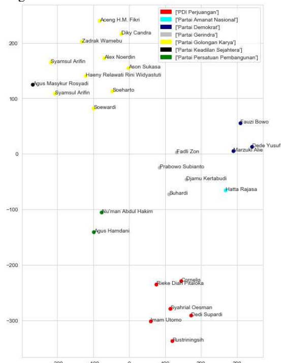
Gambar 4. Visualisasi t-SNE
