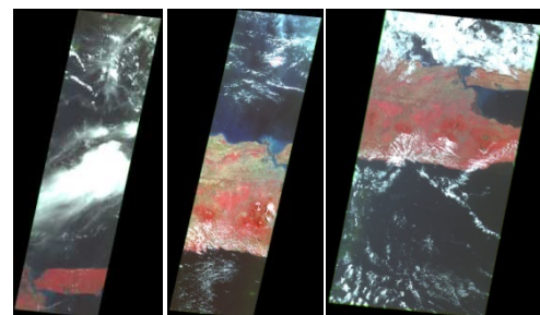
Gambar 3-6 : Citra wilayah bukit Jaddih, Madura periode 2018
