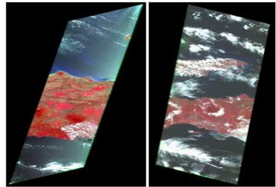
Gambar 3-5 : Citra wilayah Gunung Bromo, Jawa Timur
