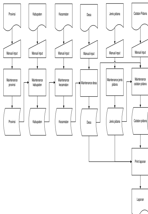
Gambar 2. System flow komputerisasi
