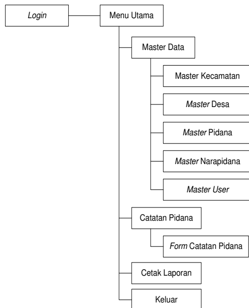
Gambar 4. Struktur Menu
