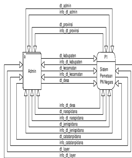
Gambar 3. Diagram Konteks
