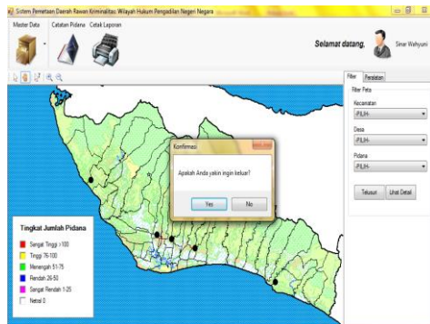
Gambar 12. Menu Keluar
