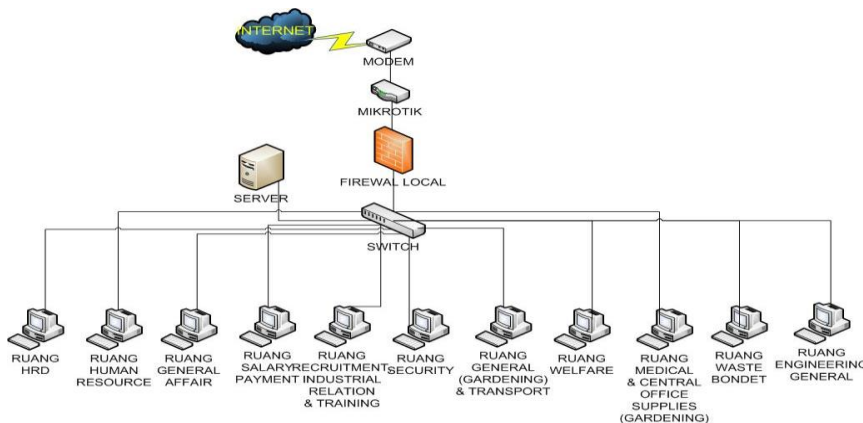
Gambar 1. Topologi Jaringan
