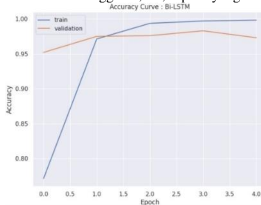
Gambar 7. Akurasi dari BiLSTM
