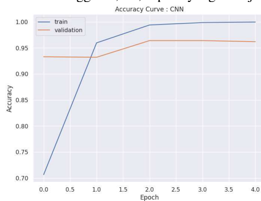
Gambar 6. Akurasi dari CNN
