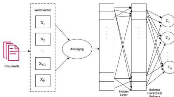
Gambar 1. Arsitektur Fasttext
