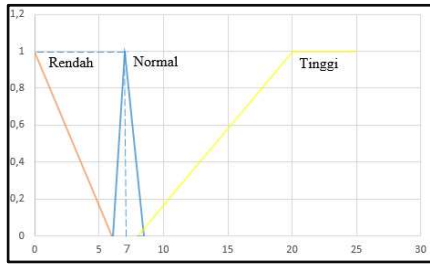
Gambar 9. Grafik variabel pH
