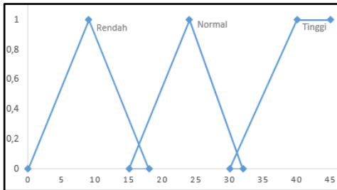
Gambar 2. Grafik keanggotaan suhu
