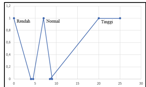
Gambar 5. grafik variabel linguistik input tds
