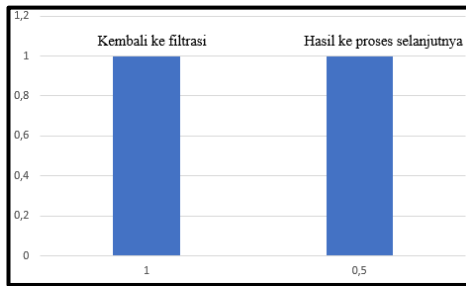
Gambar 6. grafik fungsi keanggotaan pompa air air kembali ke atas
