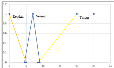
Gambar 10. Grafik variabel kekeruhan
