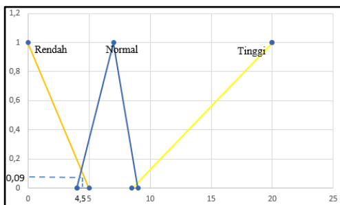
Gambar 11. Grafik variabel tds
