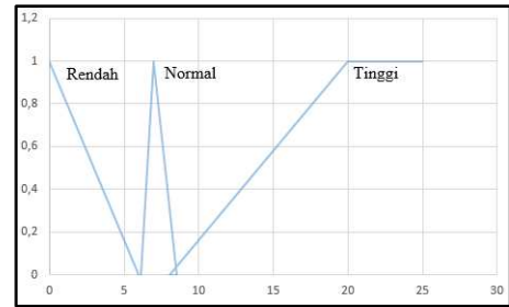
Gambar 3. Grafik fungsi keanggotaan pH
