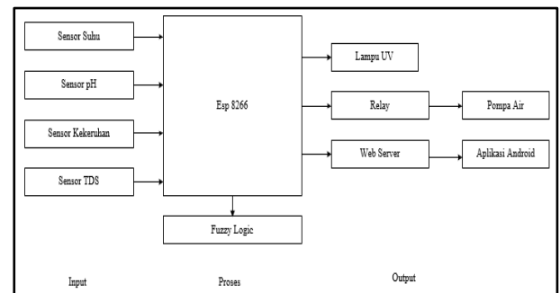
Gambar 1. Diagram blok sistem secara keseluruhan
