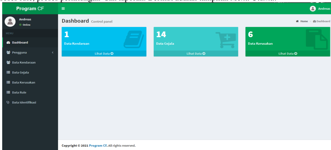
Gambar 3. Menu Utama
