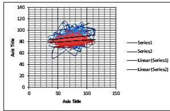
Gambar 4.4 Uji Kecocokan Model X 1 dan X 2 Terhadap Y
