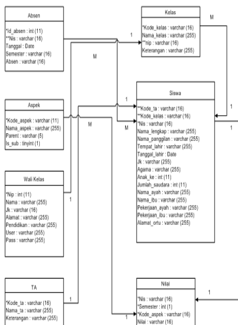
Gambar 9. Relasi Tabel
