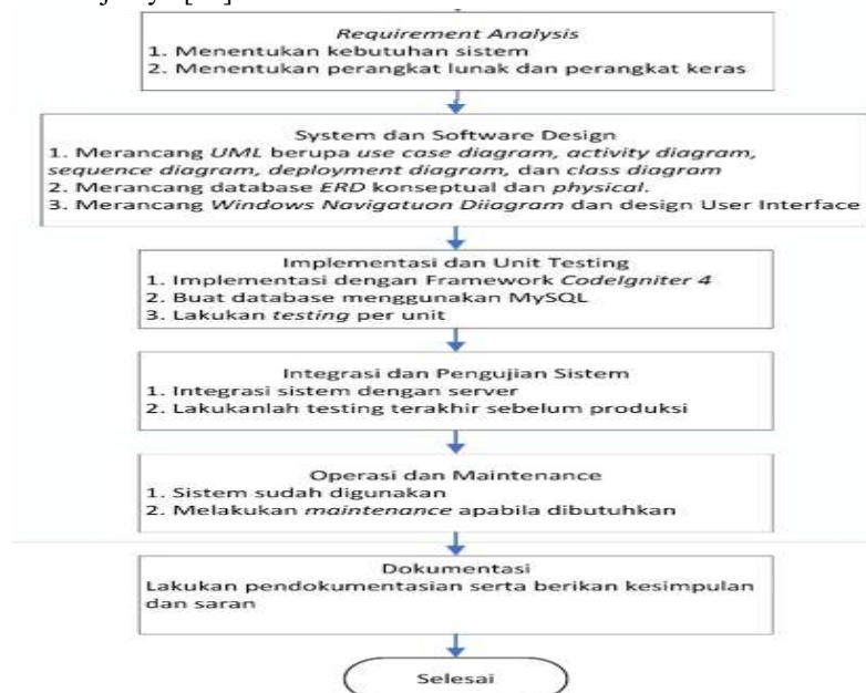
Gambar 1. Flowchart Kerangka Penelitian Sumber: Pengolahan Data (2022)
