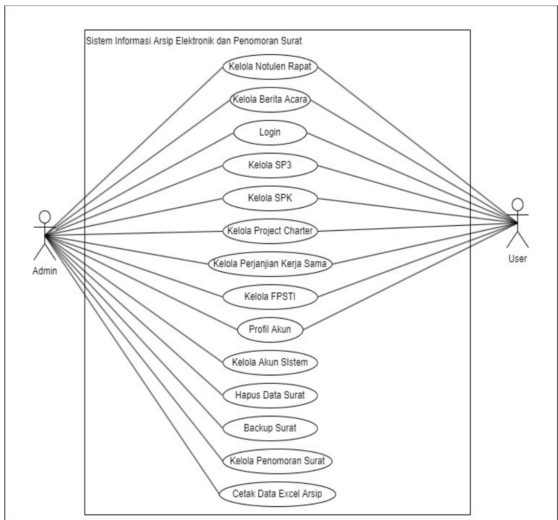
Gambar 4. Use Case Diagram Sistem Informasi Arsip Elektronik
