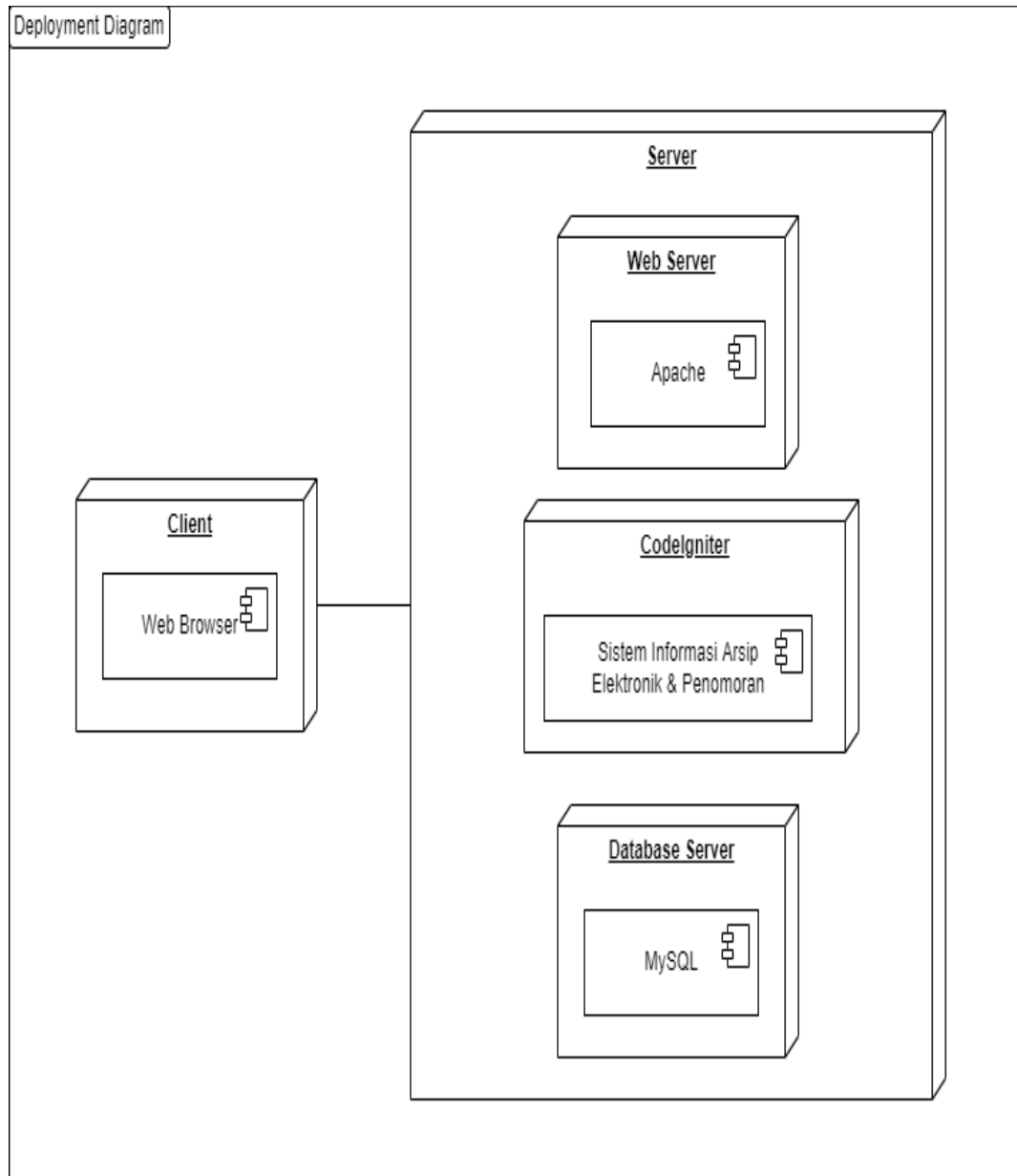
Gambar 6. Deployment Diagram Sistem Informasi Arsip Elektronik Sumber
