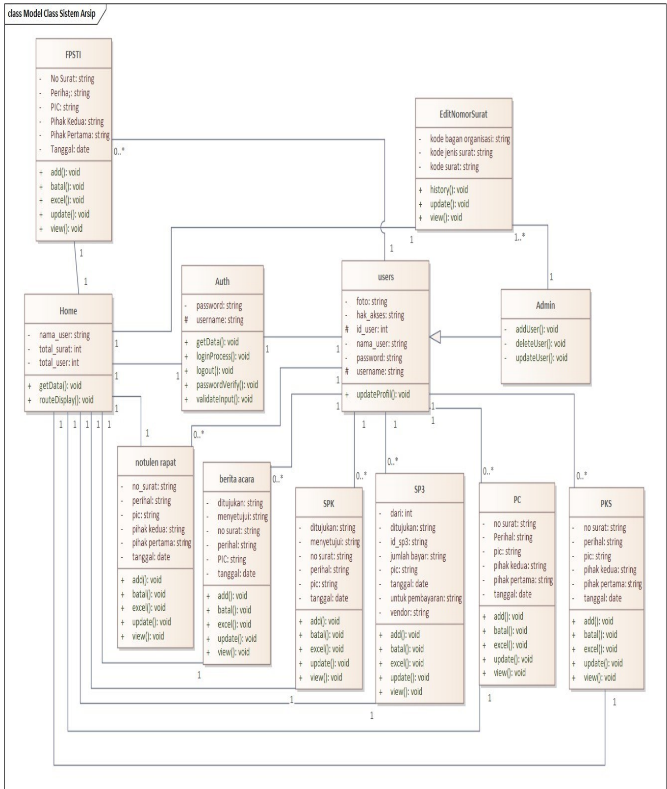
Gambar 5. Class Diagram Sistem Informasi Arsip Elektronik
