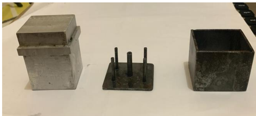
Gambar 1. Cetakan manual briket
