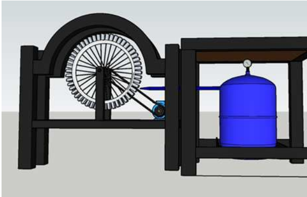
Gambar 3. Desain 3D Turbin Ipuls De Laval dengan Boiler
