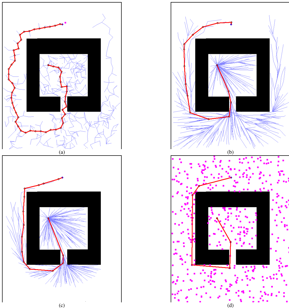
Gambar 11. Perbandingan performansi pada ruangan dengan celah sempit untuk masuk atau keluar ( trap ) :
