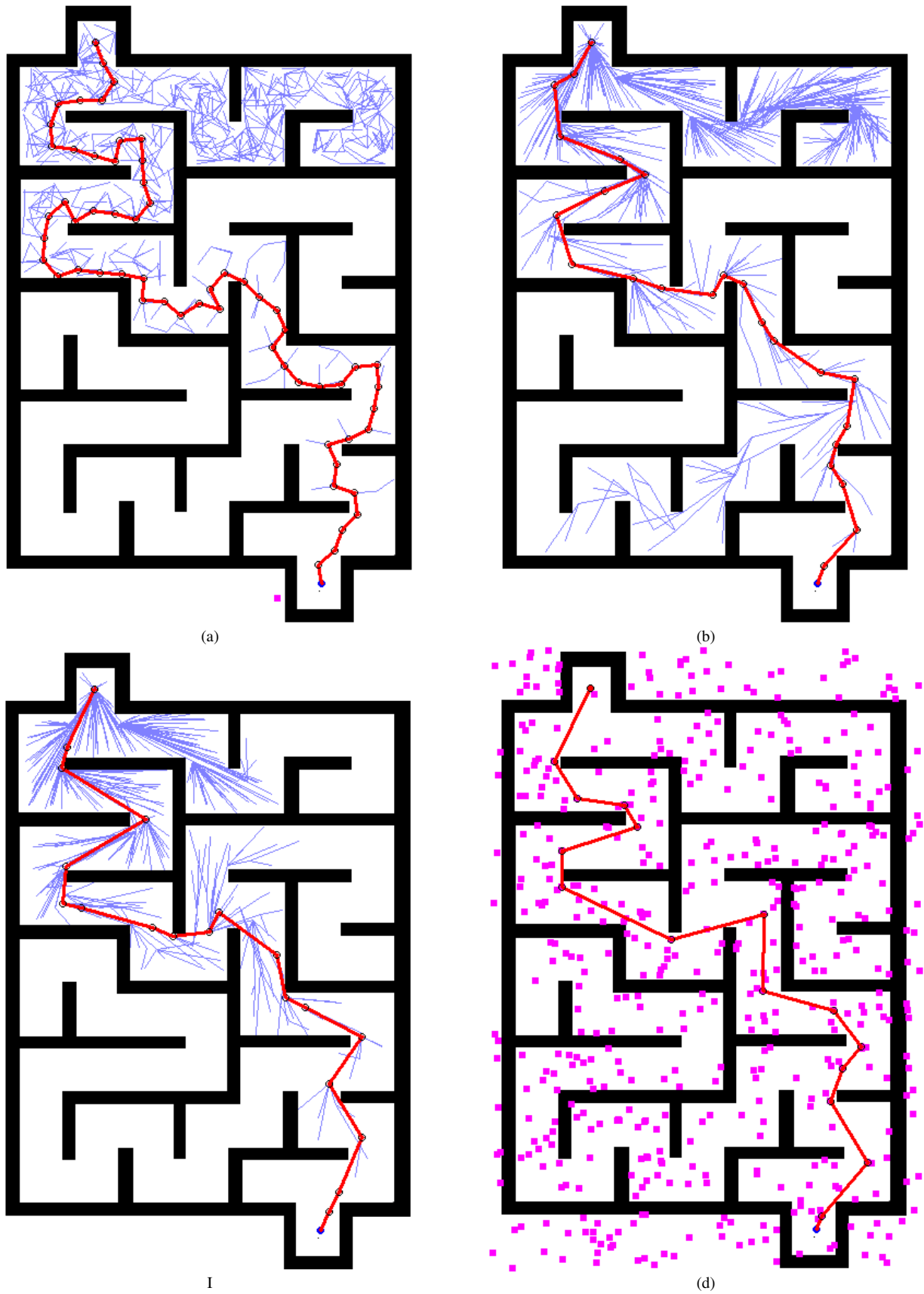
Gambar 13. Perbandingan performansi pada lingkungan labirin :
