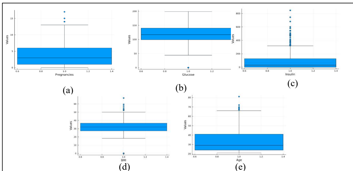
Gambar 2. Boxplot (a) Pregnancies (b) Glucose (c) Insulin (d) BMI (e) Age
