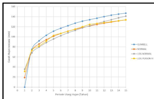
Gambar 2. Grafik Hubungan PUH dengan Curah hujan Rencana
