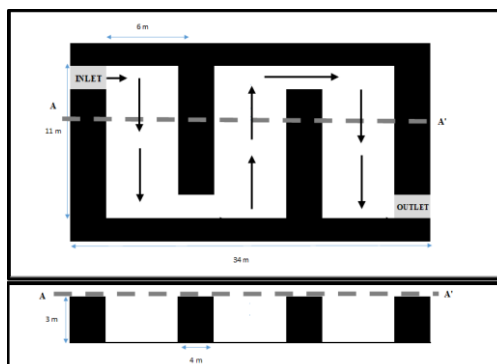
Gambar 8. Sketsa Dimensi Kolam Pengendapan
