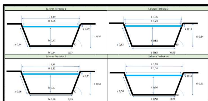
Gambar 6. Sketsa Dimensi Saluran Terbuka
