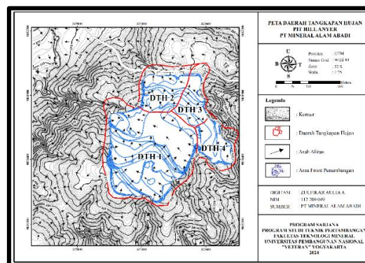
Gambar 5. Peta Daerah Tangkapan Hujan dan Arah Aliran
