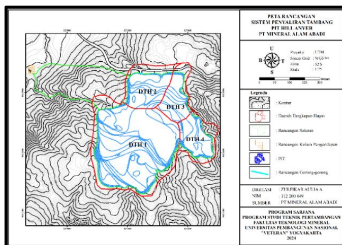
Gambar 8. Peta Rancangan Sistem Penyaliran Tambang
